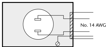
Toma bipolar con conexión a tierra
